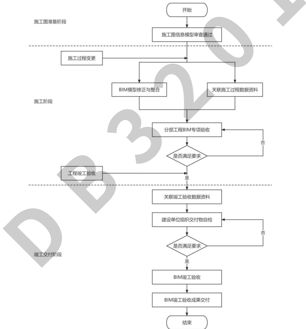
图1 竣工 BIM 形成与交付流程
